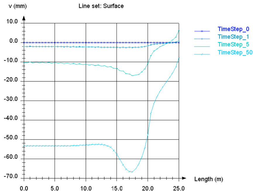
Figure 19: Evolution des déplacements verticaux sous le remblai en fonction du temps
