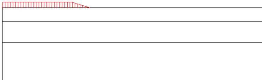
Figure 10: Distribution de la pression modélisant la géométrie et le poids de la digue
