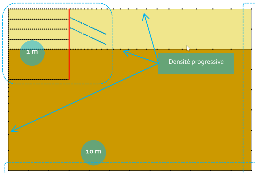
Figure 6: Zones de densités à appliquer
