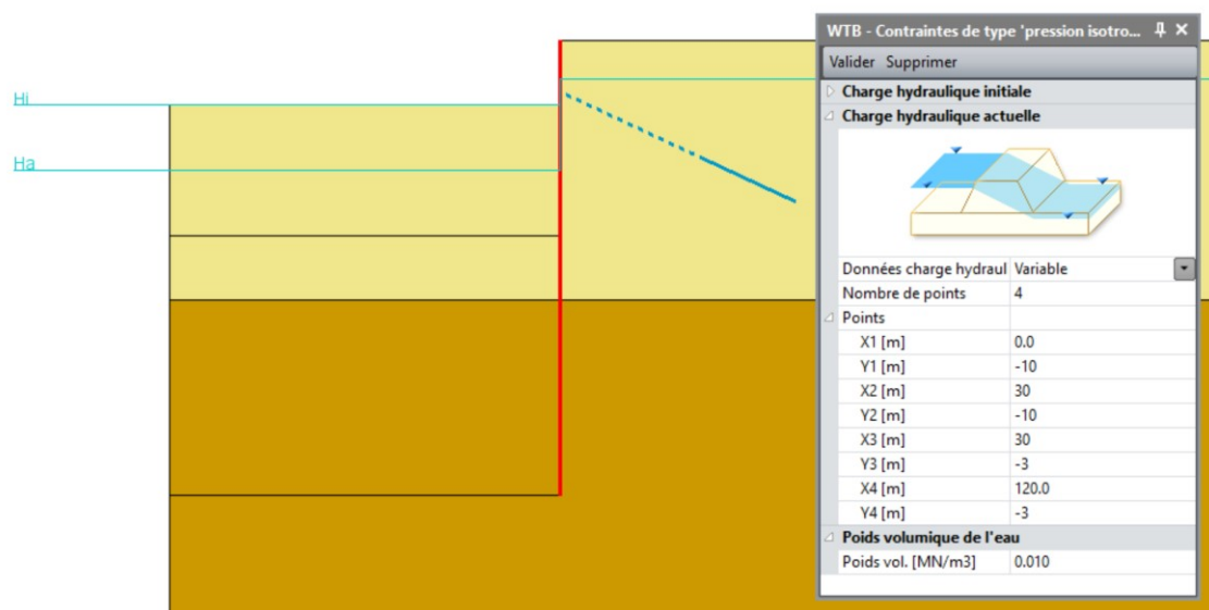
Figure 17: Rabattement de la nappe à -10 m dans l'excavation
