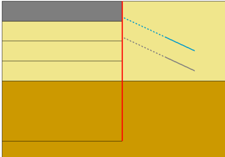
Figure 16: Statut du modèle en phase #4
