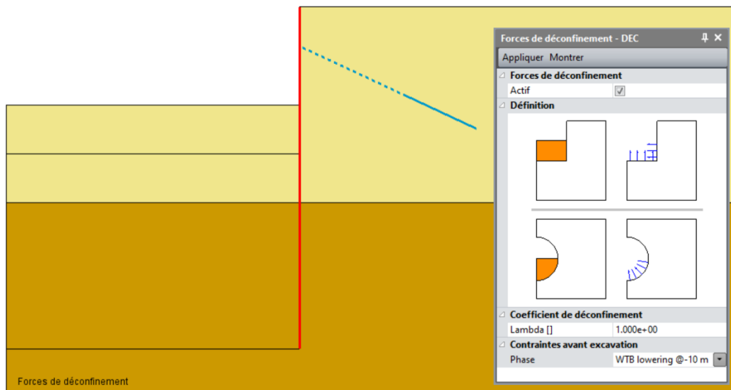
Figure 19: Définition des forces de déconfinement à -10m
