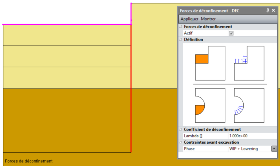
Figure 15: Définition des forces de déconfinement à -5 m
