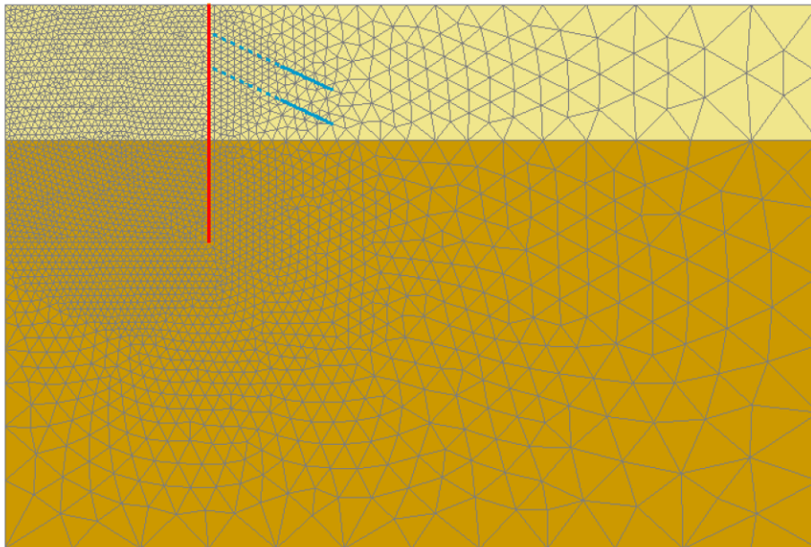
Figure 7: Vue du maillage final
