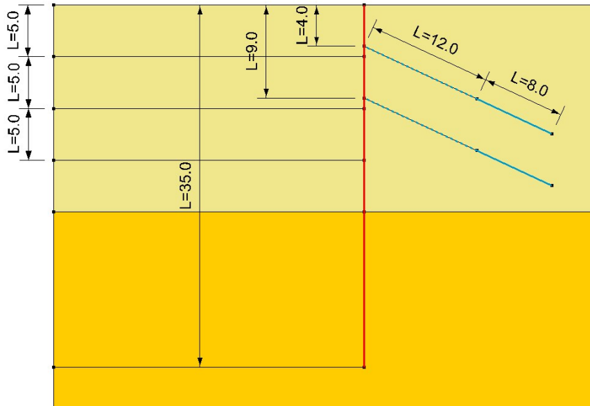
Figure 2: Zoom sur la paroi ancrée
