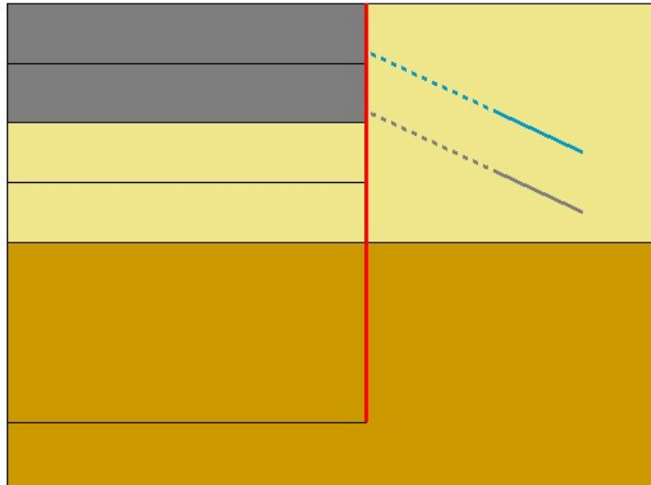
Figure 18: Statut du modèle avec les blocs en mode inactif en Phase #6
