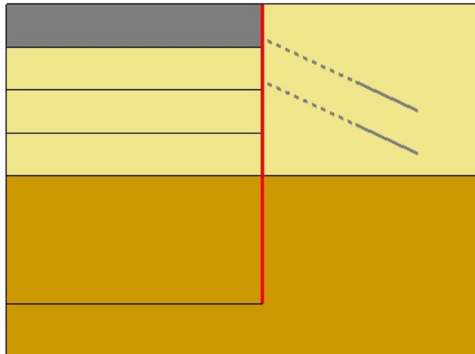
Figure 14: Statut du modèle en mode inactif en phase #3
