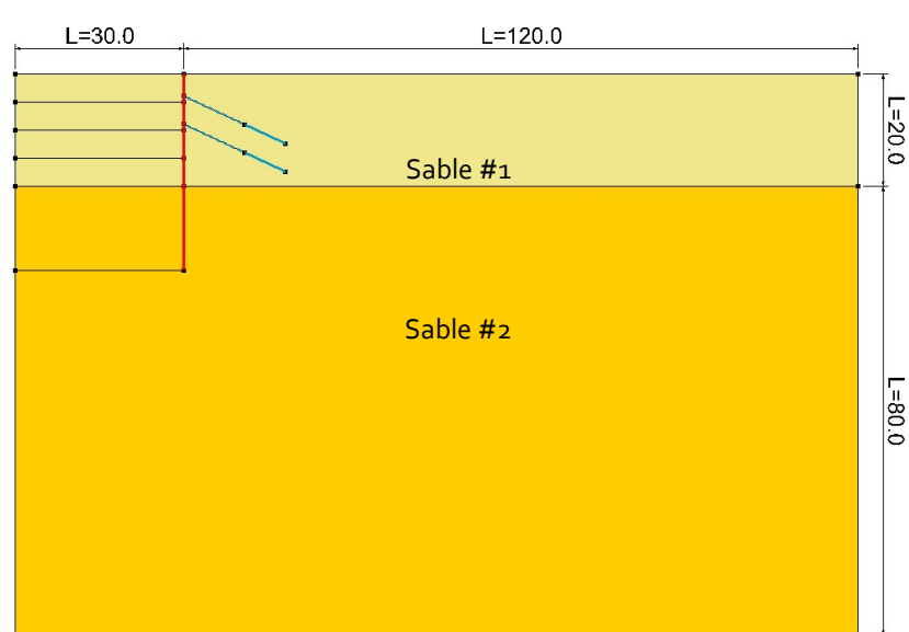
Figure 1: Modèle global (symétrie d'axe vertical en x = 0 )
